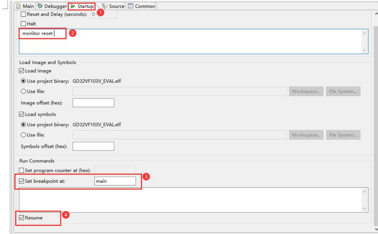
图 4.1.1.2-9 Power Writer Debugger 启动参数设置
