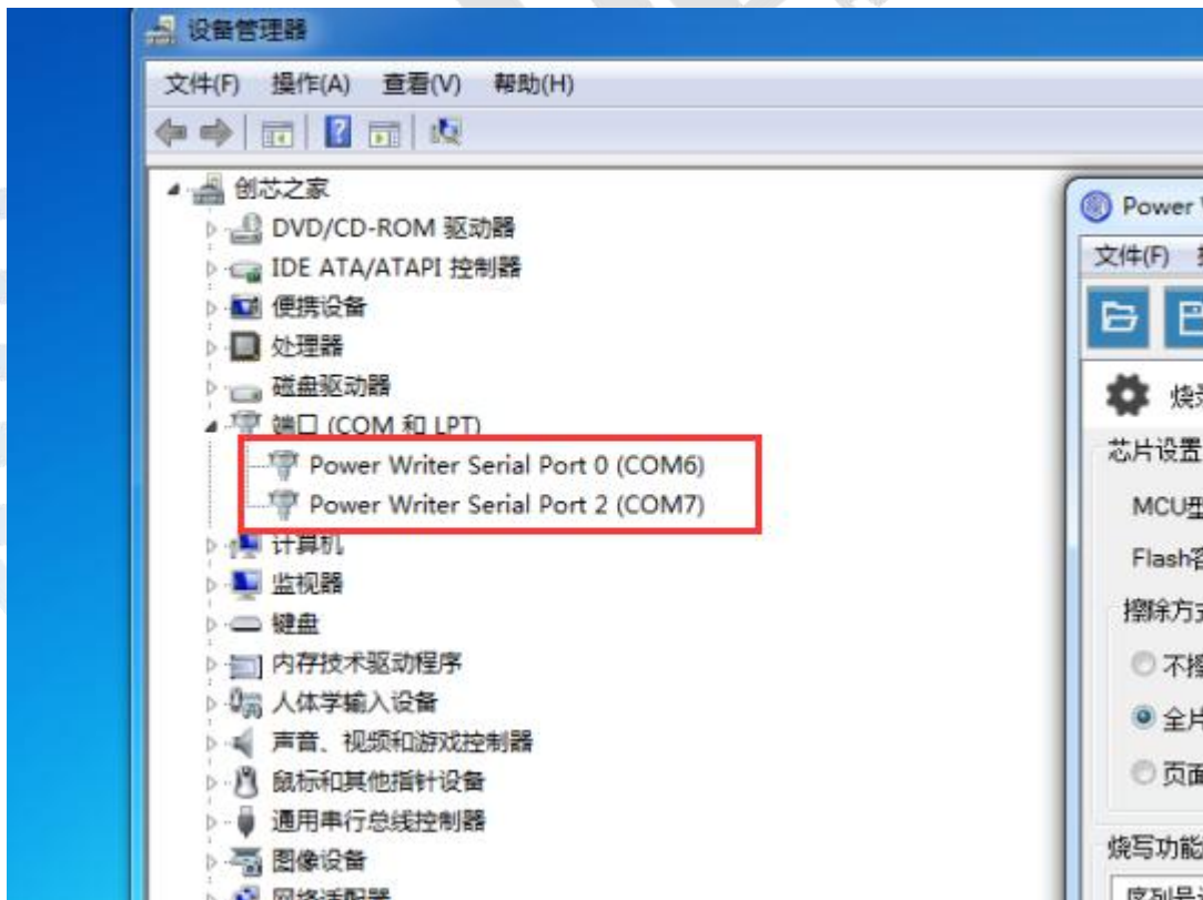
图 2.4.1.1 Power Writer For RISV 双串口以及设备路径
