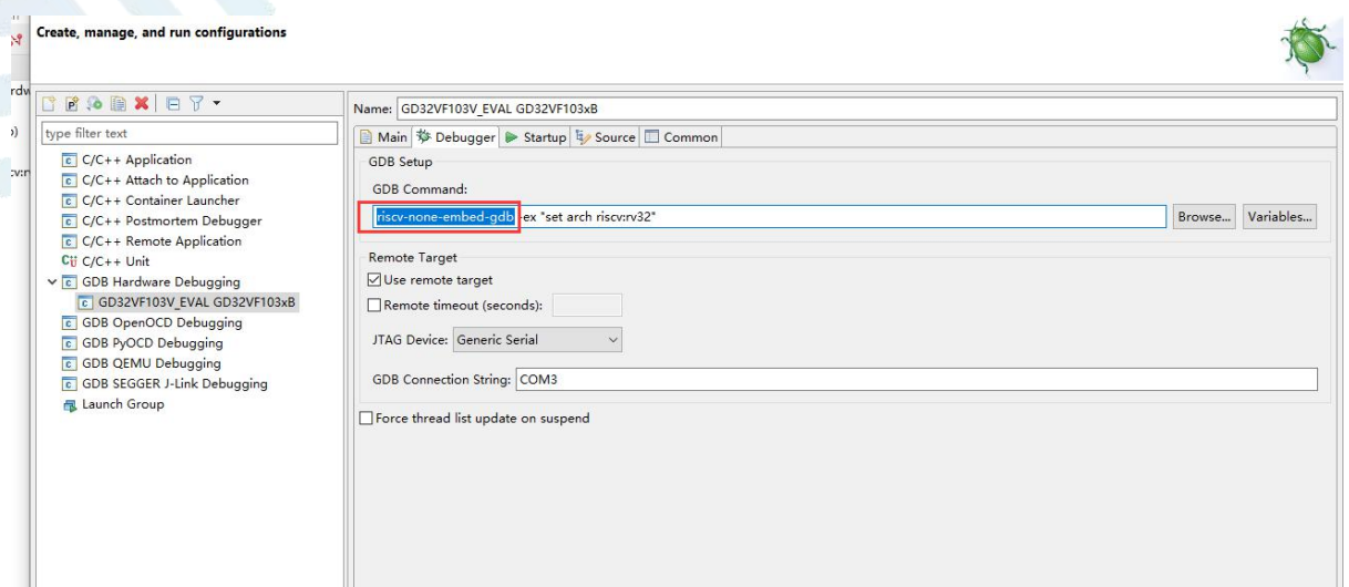
图 4.1.1.3-7 原版 eclipse + 第三方工具链 gdb 命令
