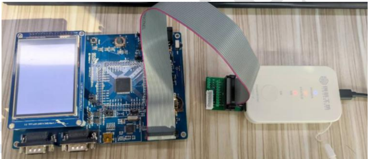
图 4.1.1.2-1 查看 Power Writer 的串行端口号并连接目标开发板
