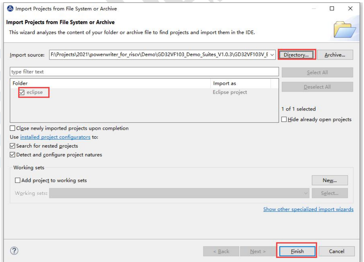
图 4.1.1.2-4 从磁盘加载项目设置
