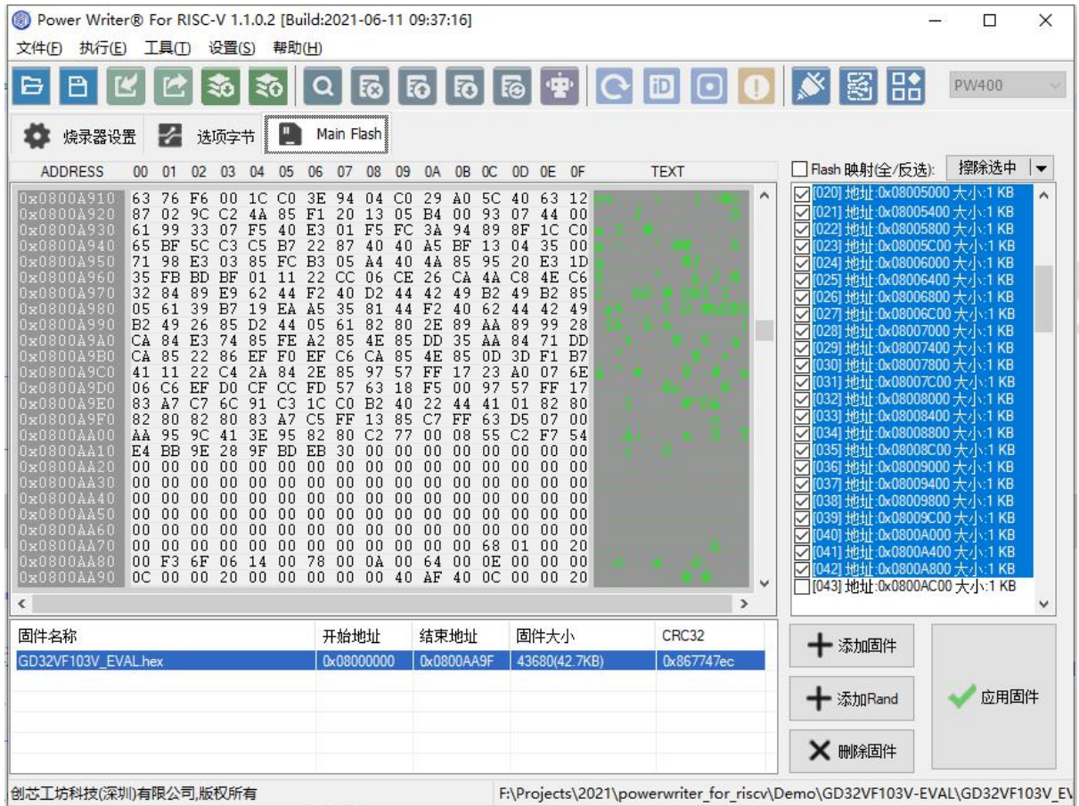
图 4.2.2-5 添加编译出的固件到 Power Writer 的 Program Memory
