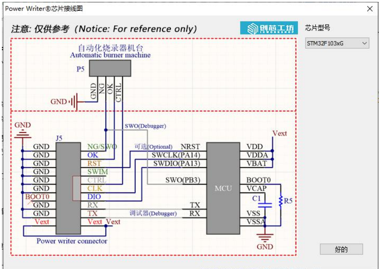
图 3.1.2.3.3 Power Writer 快速查询芯片接线图
