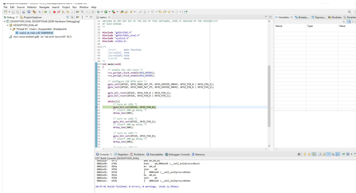
图 4.1.1.3-9 原版 eclipse + 第三方工具链 gdb 命令
