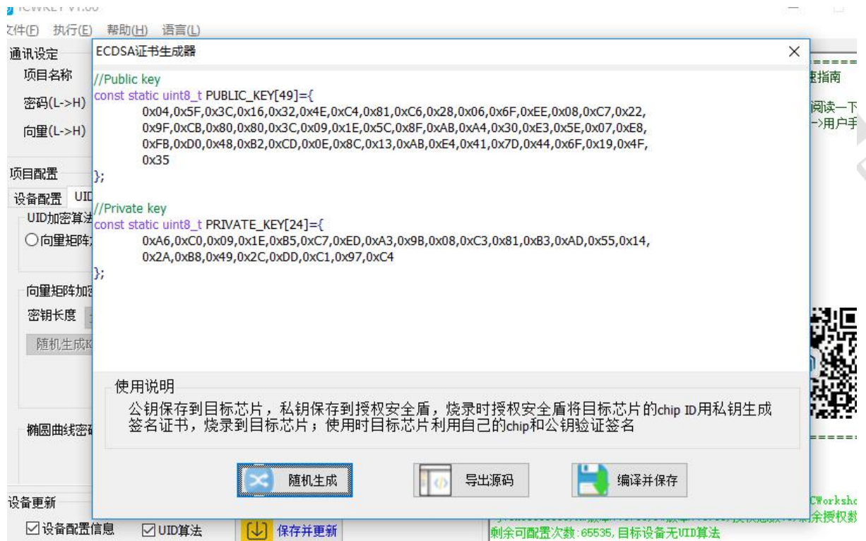
图 4.2.1.3-7 ICWKEY 配置证书
