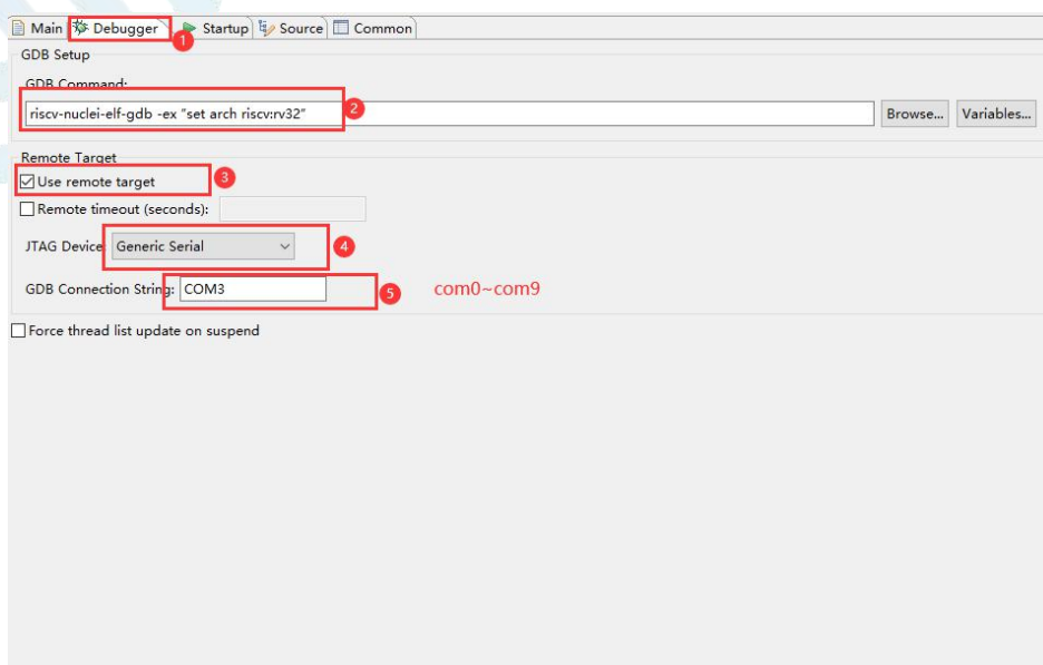
图 4.1.1.2-8 Power Writer Debugger 配置
