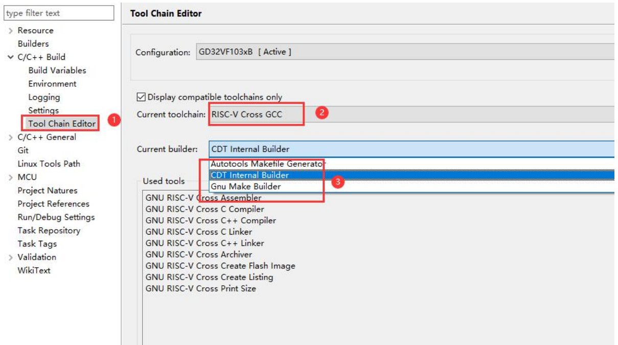
图 4.1.1.3-5 当前选择的工具链，以及 Builder 选择
