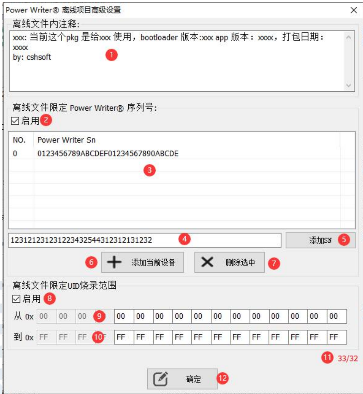
图 3.1.2.3.5 Power Writer 预留数据读写功能
